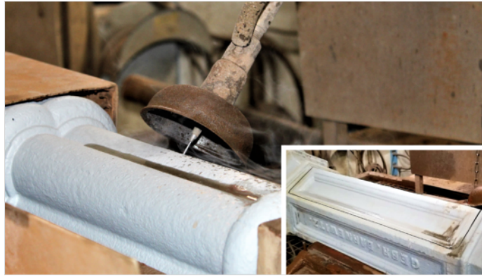
Hauseigene Roboter-Wasserstrahlanlage
